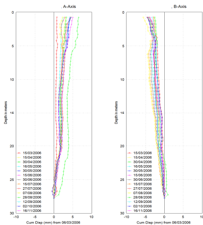
Figura 10. Gráfico de desplazamientos acumulados obtenidos de medición inclinométrica
