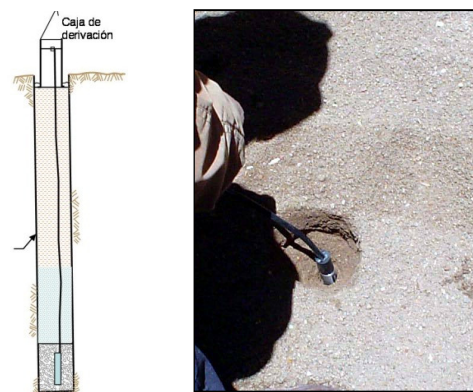
Figura 5. Instalación de piezómetro eléctrico de cuerda vibrante
