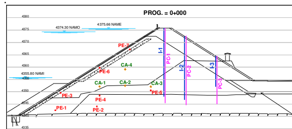
Figura 1. Ubicación de piezómetros, celdas de asentamiento e inclinómetros en la Sección 1-1 de la presa Pillones
