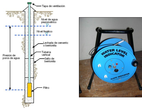
Figura 4. (a) Instalación de piezómetro tipo Casagrande (b) Indicador de nivel de agua
