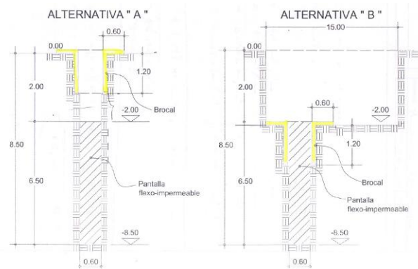
Figura 6. Alternativas para construcción de pantalla
