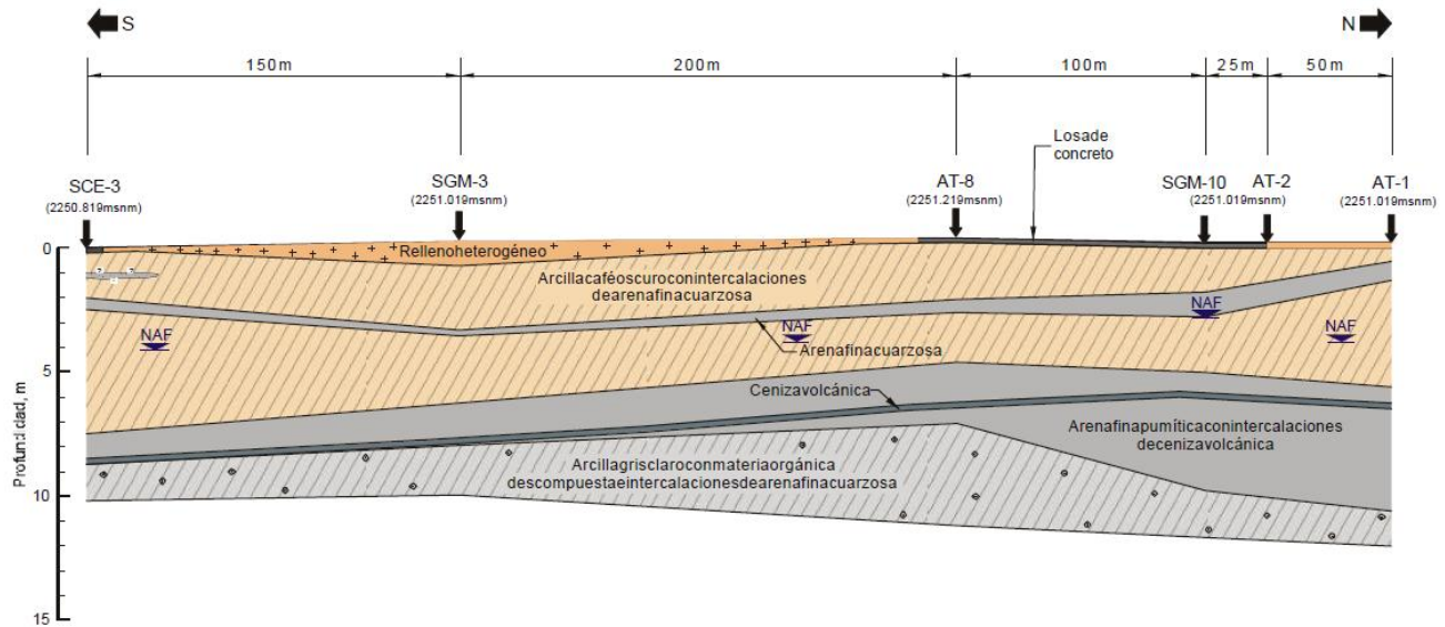
Figura 4. Perfil estratigráfico del sitio
