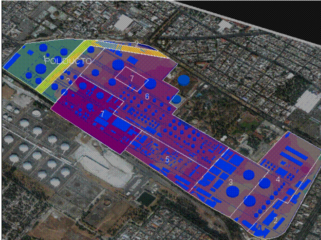
Figura 2. División de áreas consecuencia de la caracterización de suelos.
