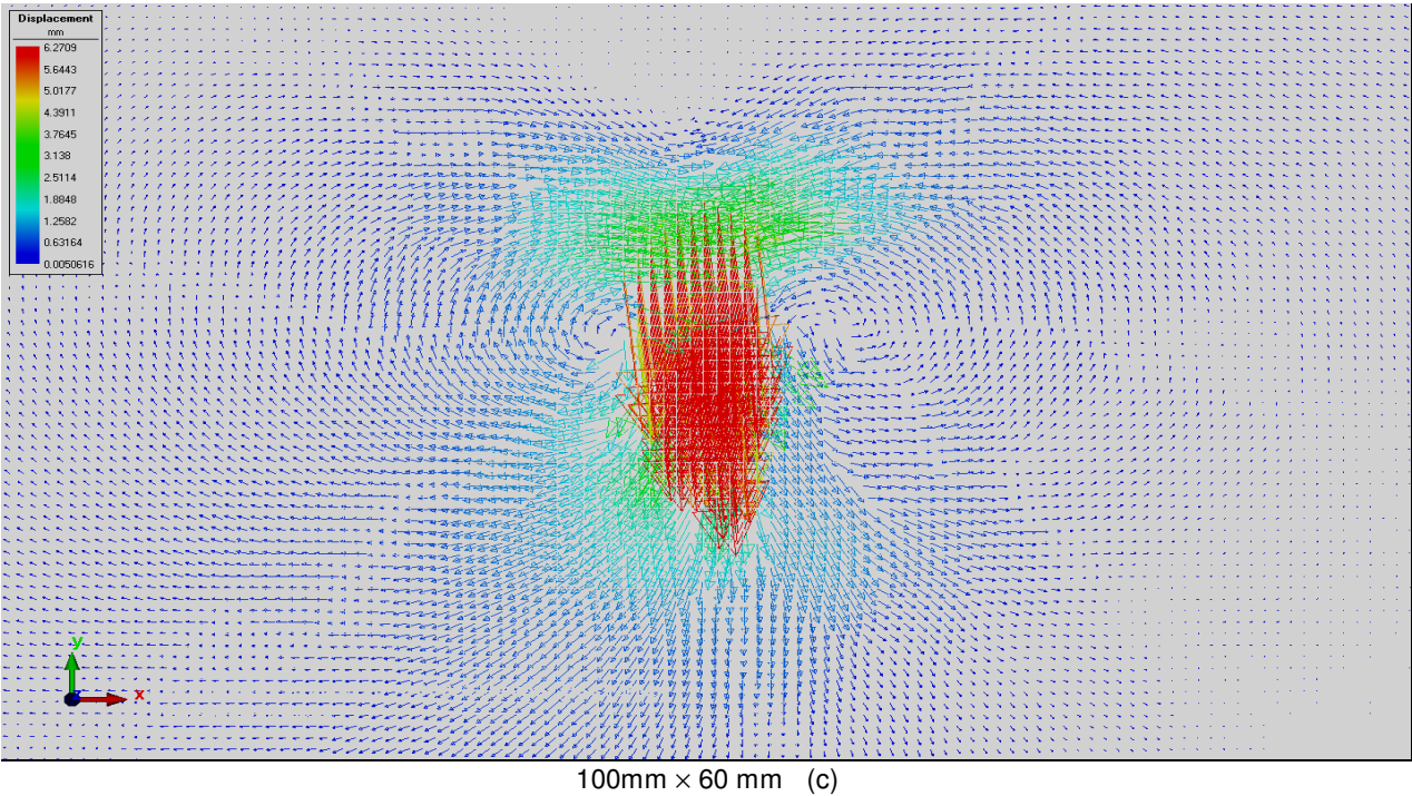
Figura 14. Resultados de la aplicación de la correlación de imágenes digitales DIC para las fotografías tomadas durante la penetración del mini T-bar_Visu03 a la profundidad de z/D = 26.1 . Superposición de las dos imágenes analizadas, de referencia y a correlacionar (a), curvas de isovalores de los vectores de desplazamientos en mm (b), y vectores de desplazamientos (c).
