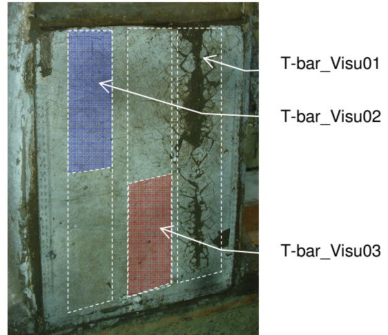
Figura 10. Posición de los ensayos de penetración mini T-bar para la visualización del mecanismo de falla.
