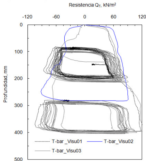
Figura 11. Serie de ciclos aplicados en los ensayos de penetración del min T-bar en un suelo arcilloso de aguas profundas. Ensayos Visu01, Visu02 y Visu03.
