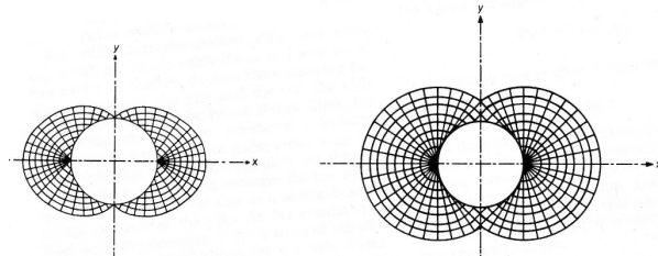
Figura 2. Redes de curvas características para una superficie lisa (a) y rugosa (b), Randolph y Houlsby (1984).
