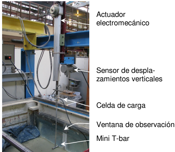
Figura 4. Sistema para la penetración del mini T-bar.
