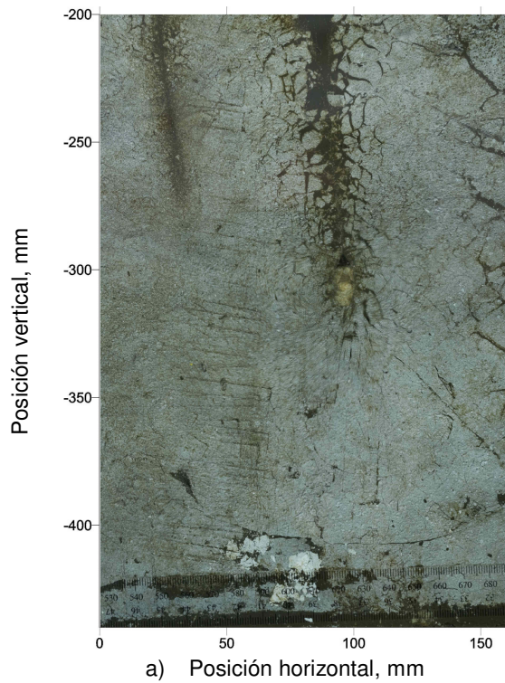
Figura 13. Resultados de la aplicación de la correlación de imágenes digitales DIC para las fotografías tomadas durante la penetración del mini T-bar_Visu02 a la profundidad de z/D = 2.2 . Superposición de las dos imágenes analizadas, de referencia y a correlacionar (a), curvas de isovalores de los vectores de desplazamientos en mm (b), y vectores de desplazamientos (c).
