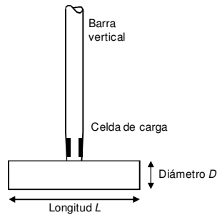
Figura 2. Penetrómetro tipo T-bar o full-flow.
