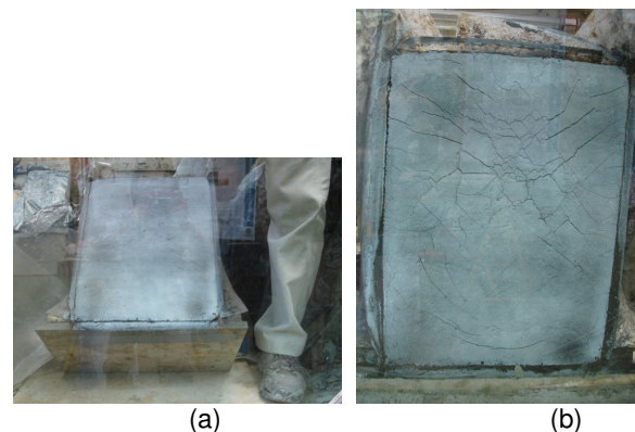
Figura 8. Instalación del bloque de suelo al interior del tanque (a), superficie del bloque de suelo al contacto con el vidrio (b).
